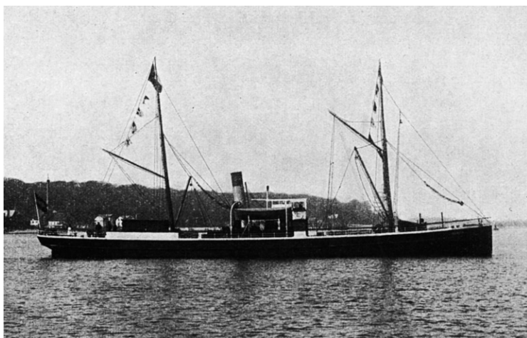
Abb. 5 Charterdampfer HOLSATIA als Fischereiforschungsschiff, 1901. (Aus: Die Ostsee-Expedition 1901 des Deutschen Seefischerei-Vereins . [= Abhandlungen des Deutschen Seefischerei-Vereins , Bd. VII]. Berlin 1902, S. IV)
