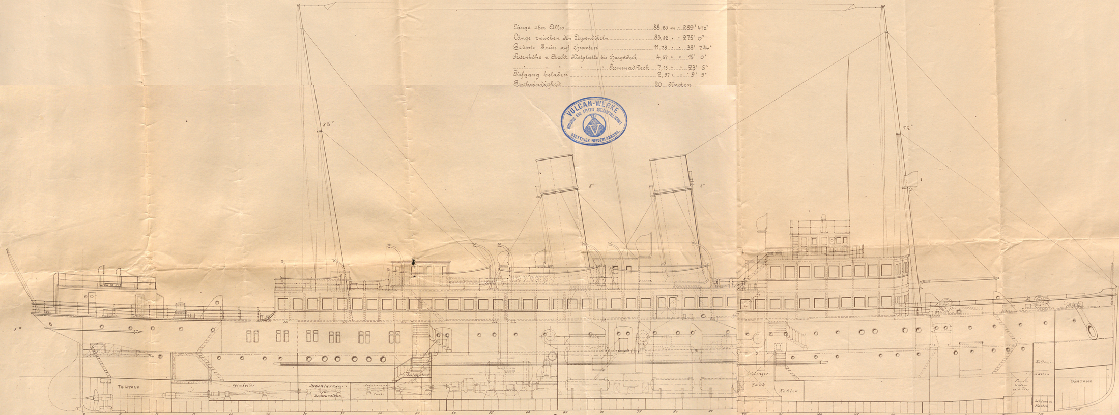
Längsschnitt.
